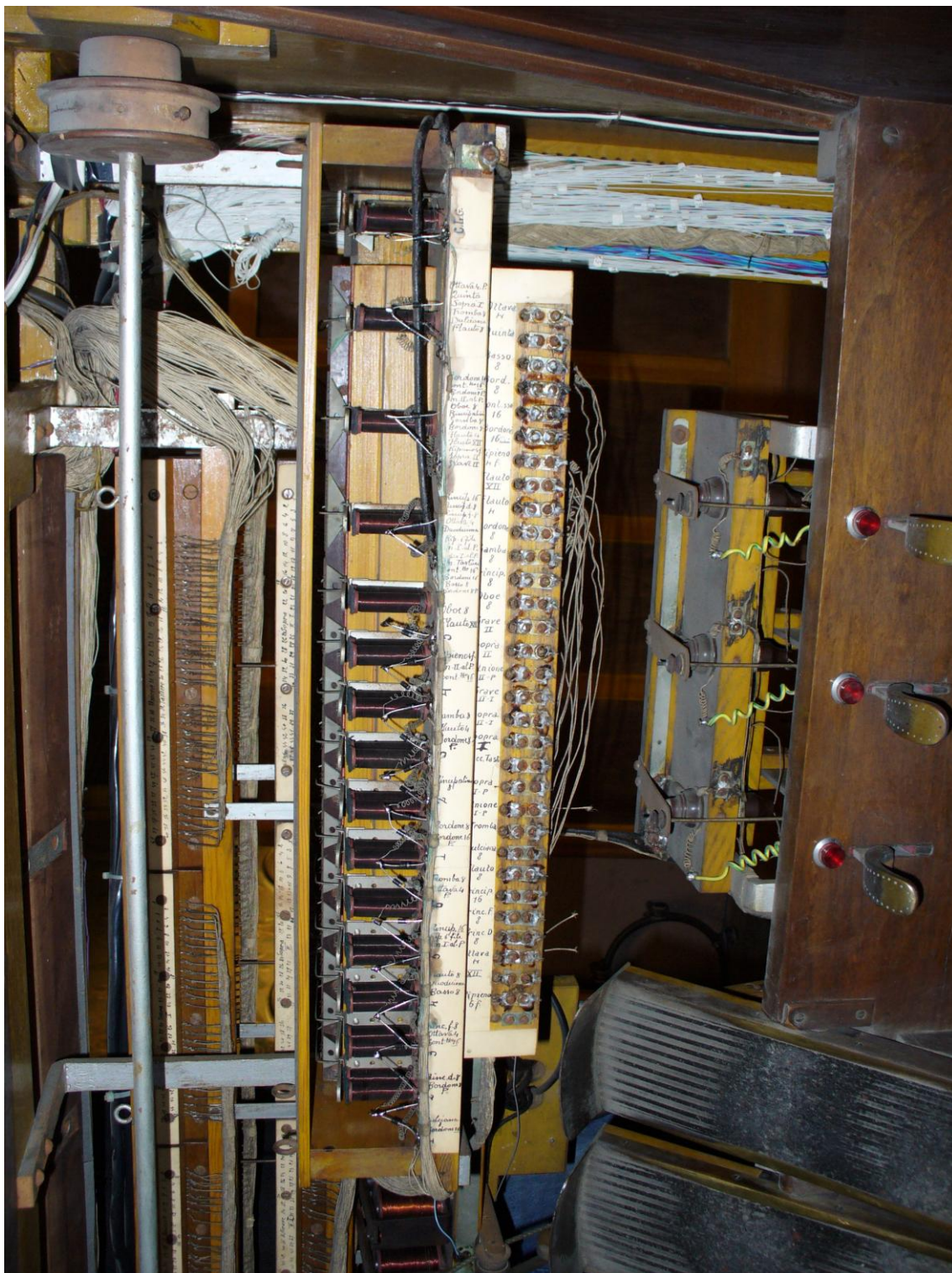
Particolare dei diodi installati sugli elettromagneti delle Combinazioni Fisse Foto 12/15
