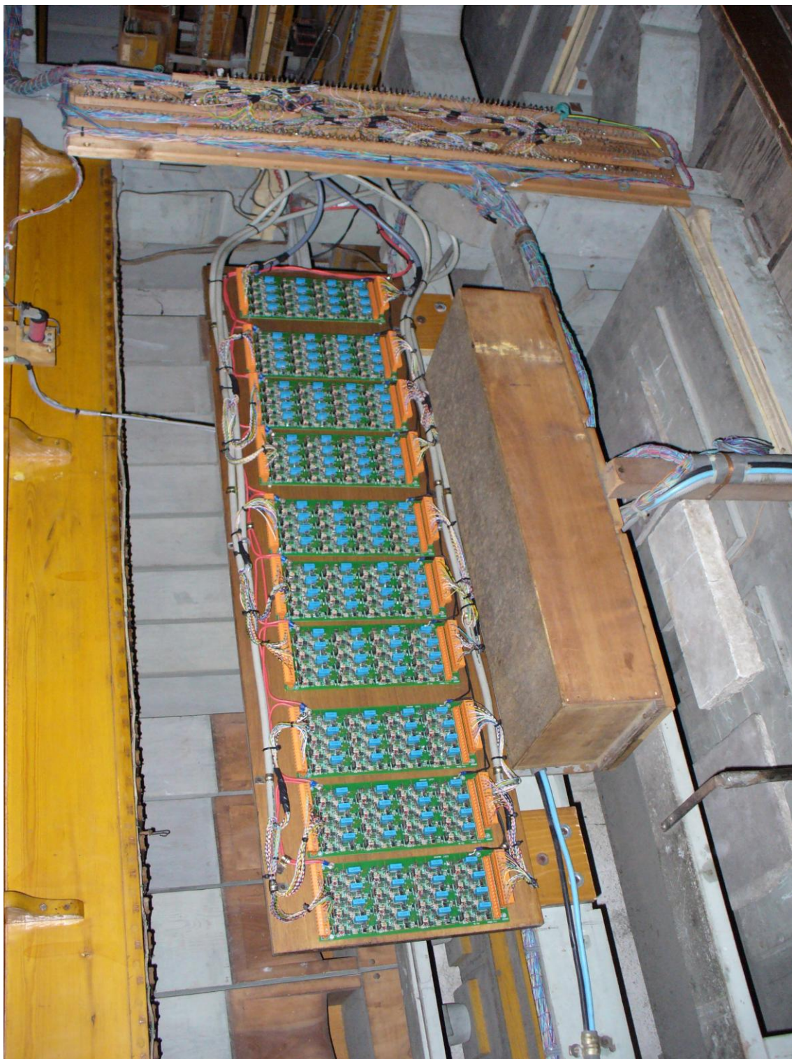
Tutte le schede montate e cablate definitivamente
