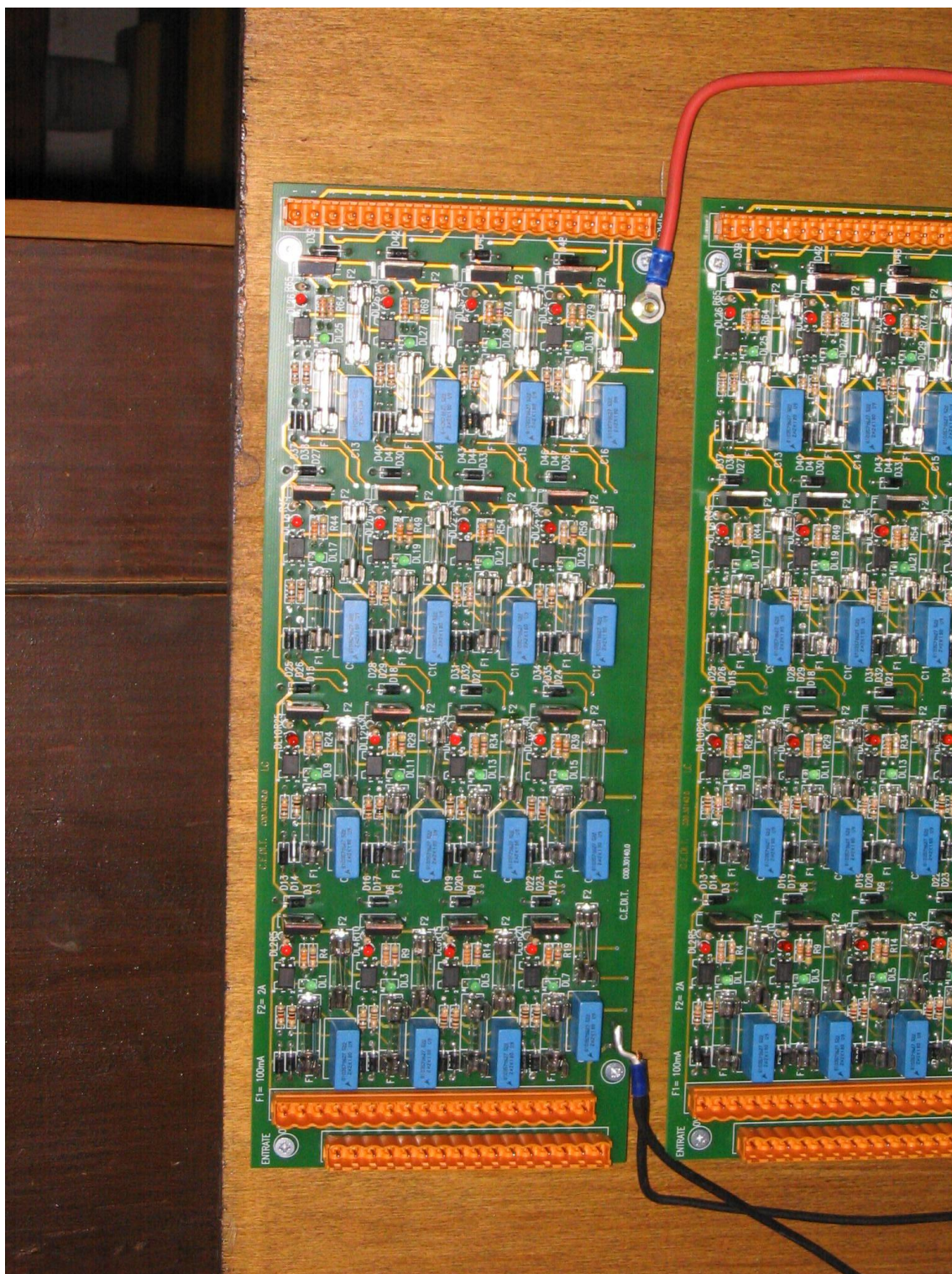
Particolare delle schede prima del cablaggio definitivo
