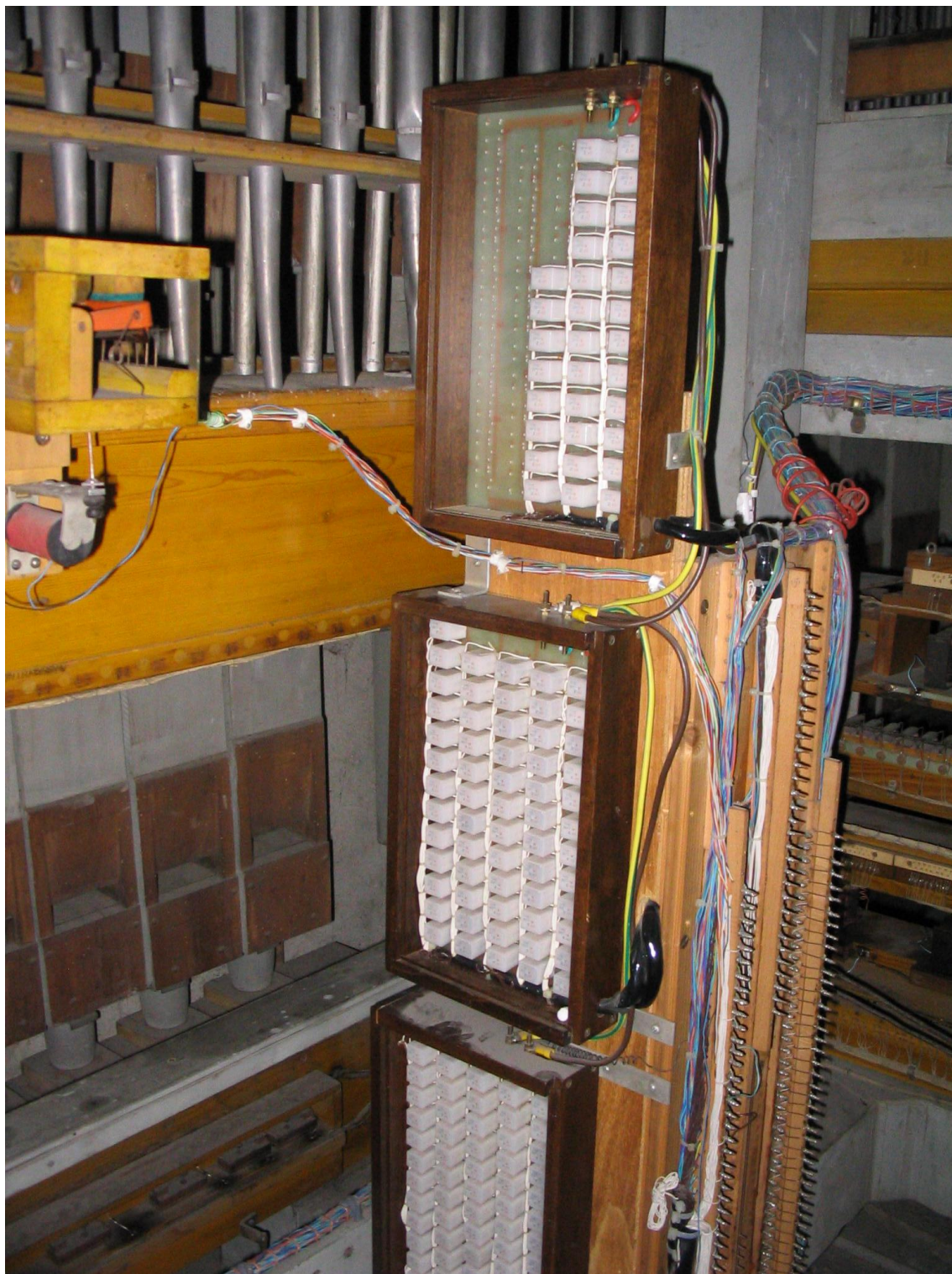
Cassettine (aperte) contenenti i microrelé e la rastrelliera di interfaccia.
