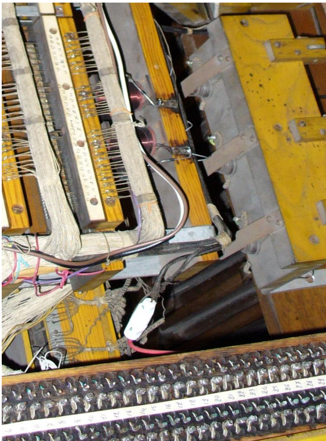
Particolare dei diodi installati sui "relé multipli a pettine" delle Unioni e del fusibile di protezione per le Combinazioni Fisse
