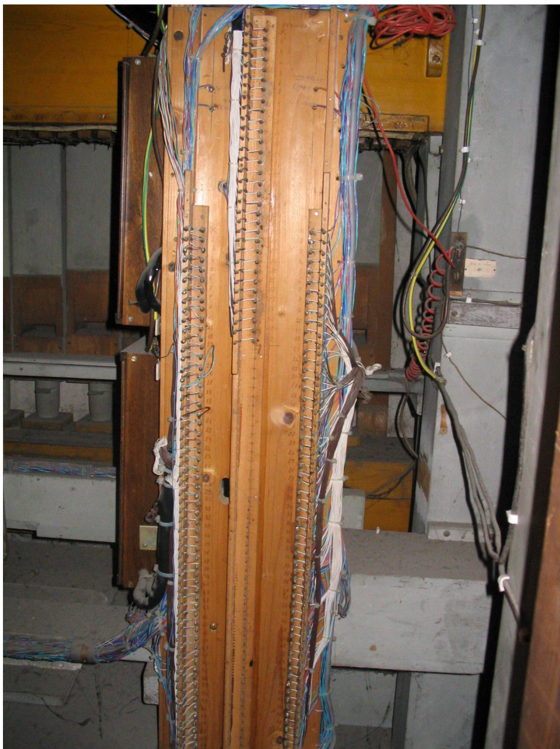
Cablaggi dei microrelé da e per la rastrelliera di interfaccia.
