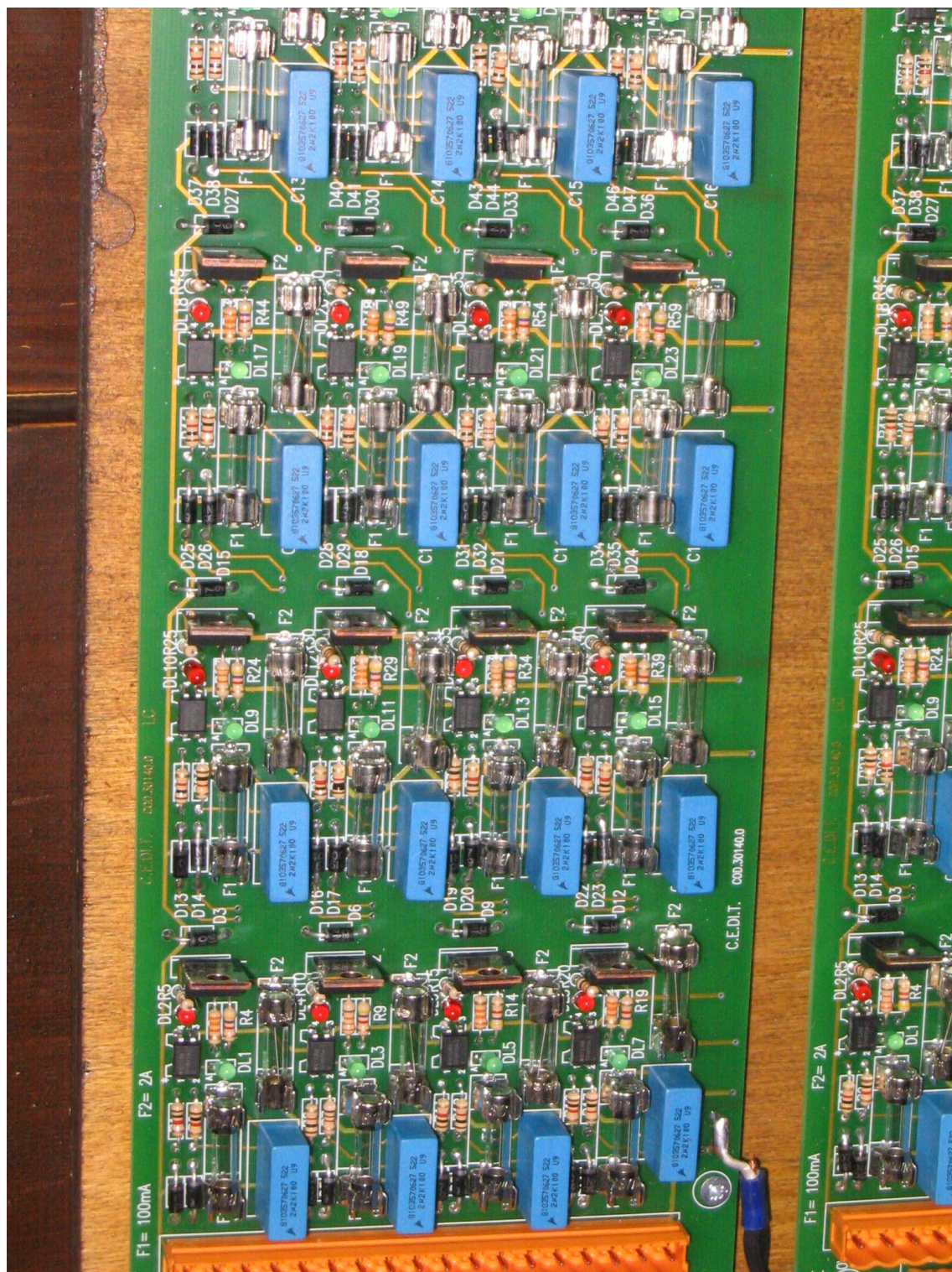
Particolare di una delle schede prima del cablaggio definitivo
